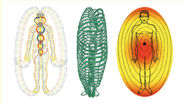
Longlines Ost-West-Ströme Spiralströme
