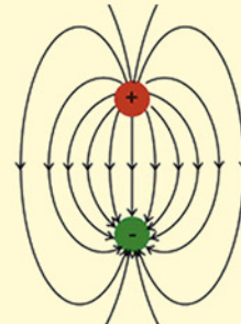
Elektromagnetisches Feld
